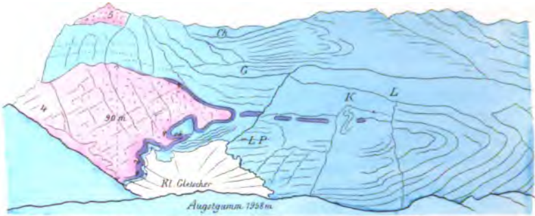
Fig. 1. Endigung des Hauptgneisskeils 4 am Gstellhorn, oberhalb der Alp Augstgamm. Ch - Choresches, G - altes Gletscherbett, K - Känzell, L - Leiteren, LP - Losterplatten.
